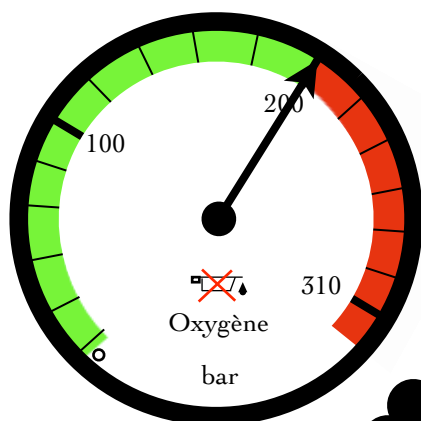
Manomètre indiquant la pression dans la bouteille d'oxygène. (Pression de stockage d'une bouteille 200 bar)
