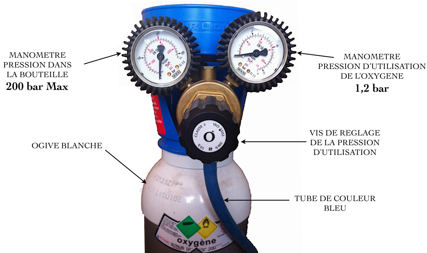
Manomètre indiquant la pression dans la bouteille d'oxygène. (Pression de stockage d'une bouteille 200 bar)
